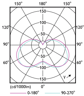
LED Candle B35 4,9W E14 827 FR
